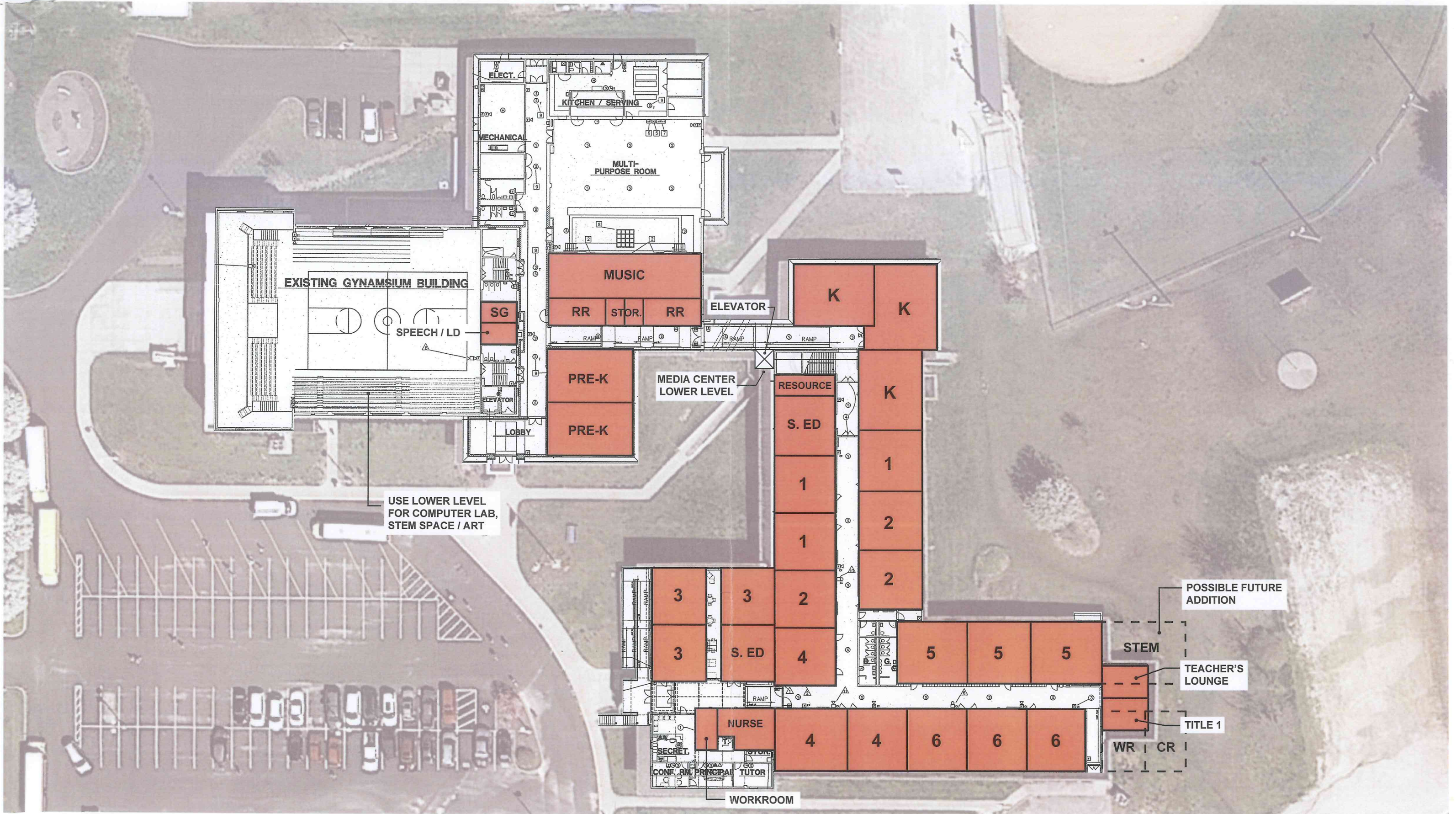
NE DUBOIS PRE K - 6 SCALE 1" : 40' - 0"
